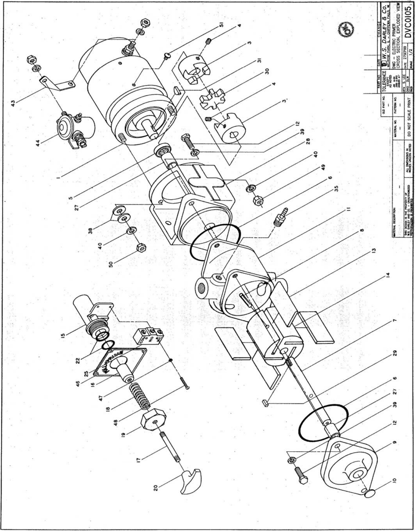
电动真空泵维修装配参考图纸
